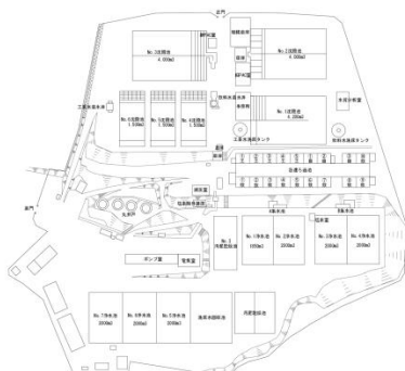
宮原浄水場全体図
