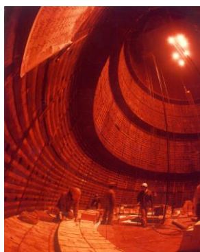
高炉内施工風景
