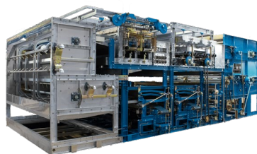
全自動海苔乾燥機械
